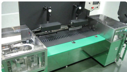
バイアル目視検査装置 (GMP対応)
