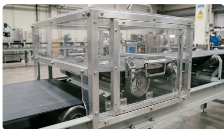
安全カバー (透明・内部視認)
